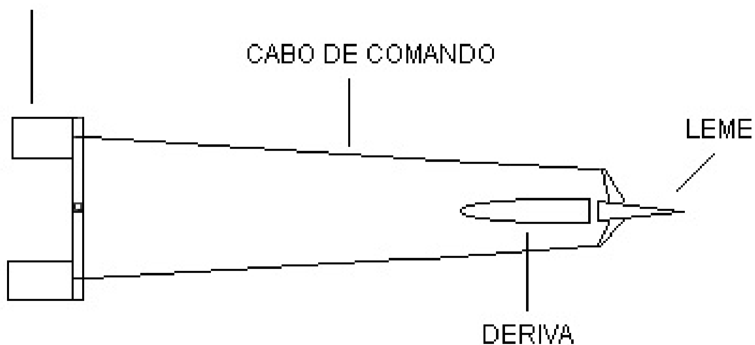
Figura 4.15 - Comando do leme
