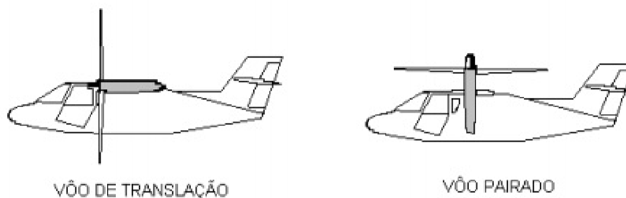
Figura 4.2 - Converteiplano
