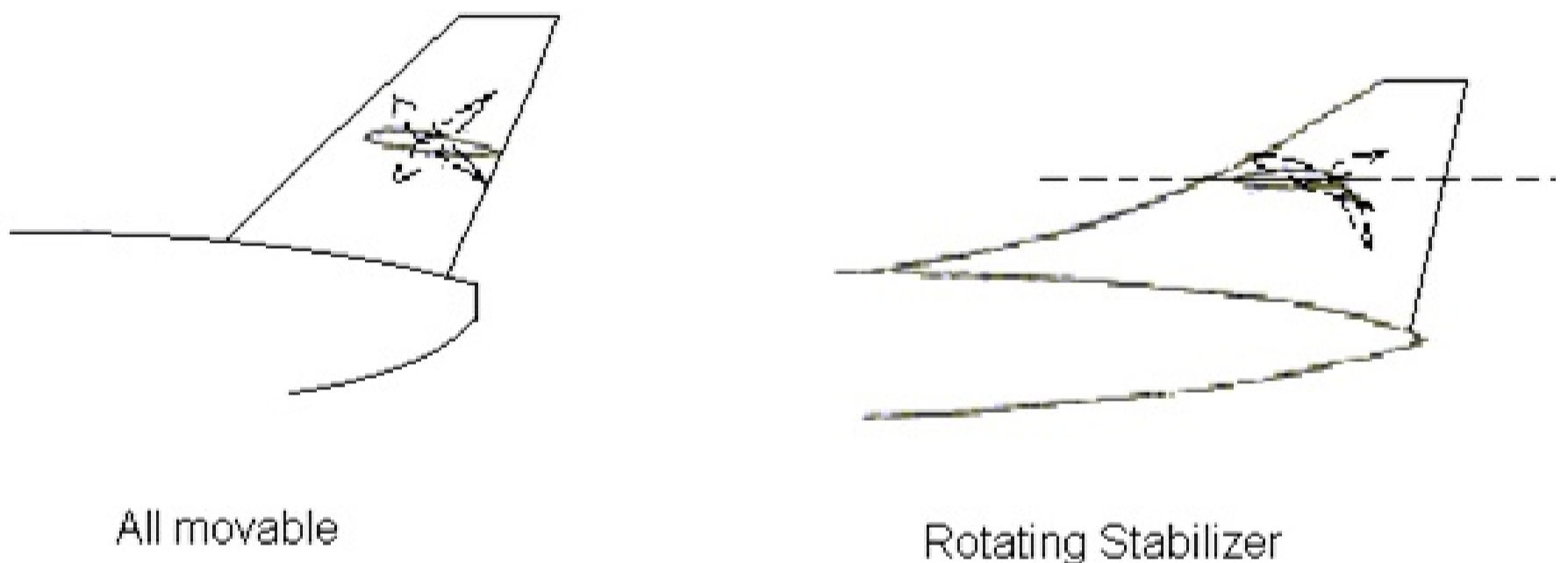
Figura 4.9 - Empenagens
